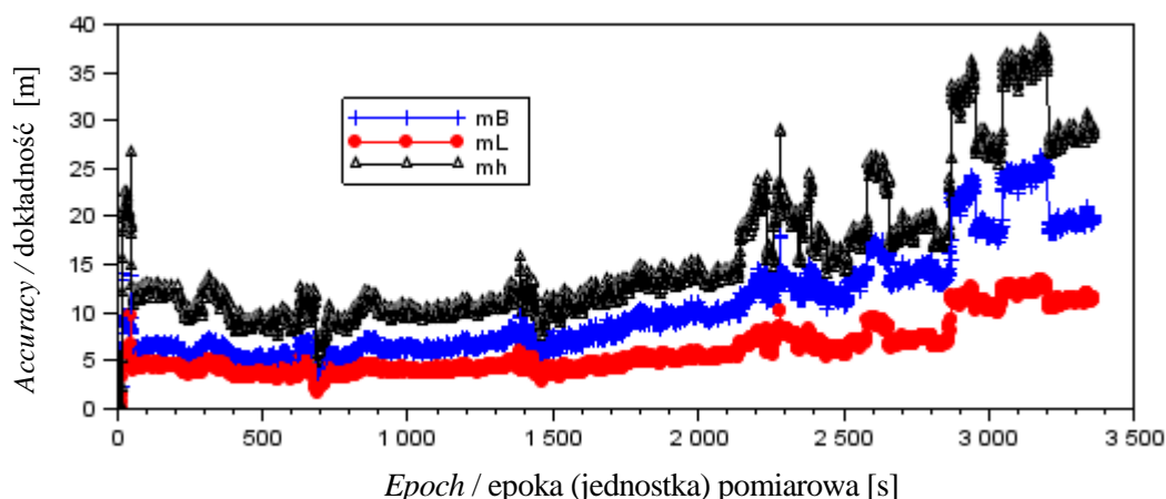
Rys. 6. Dokładność współrzędnych samolotu Cessna 172 w układzie geodezyjnym BLh Źródło: opracowanie własne Fig. 6. Accuracy of co-ordinates for Cessna 172 plane in geodetic system BLh Source: own development
